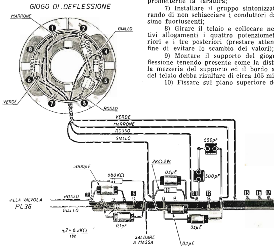
Fig. 22 - Cablaggio giogo deflessione e bassetta B
