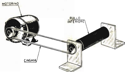
Fig. 5. - Trasmissione di moto con sistema a cinghietta.
