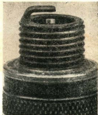
Fig. 4 - A grado termico esatto, la corrosione degli elettrodi — dopo 1000 chilometri di marcia — risulterà minima. Nel caso l'elettrodo risulti consumato eccessivamente apparirà evidente come la candela montata sia di tipo troppo caldo.
