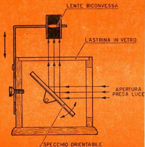
Fig. 4 - Sezione di microscopio semplice.
