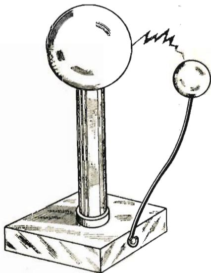
Fig. 14. - Il generatore VAN DE GRAAFF può considerarsi pure un generatore di ozono. All'uopo procederemo a sostituire il dozzinale mestolo in alluminio con una sfera metallica cava.
