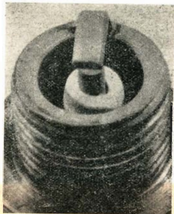
Fig. 9 - Verificandosi screpolature o ammanchi di ceramica nell'isolante, balzerà evidente come la candela utilizzata risulti troppo calda, per cui si procederà alla sua sostituzione con altra più « fredda ».
