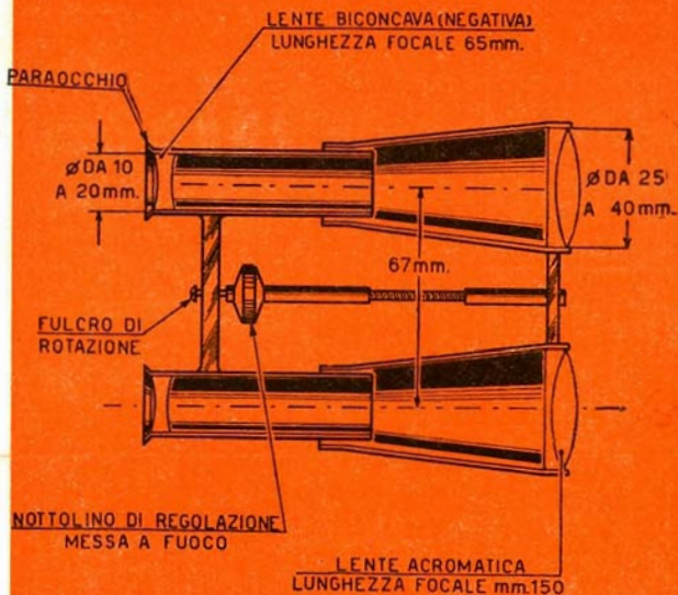
Fig. 8 - Binocolo da teatro sezionato.
