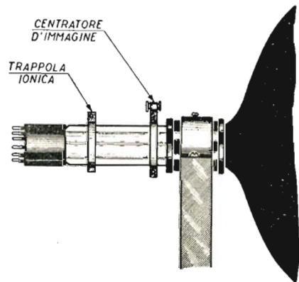
Fig. 24 - Sistemazione centratore d'immagine e giogo di deflessione
