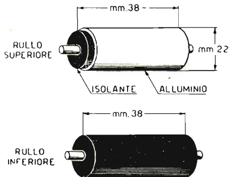
Fig. 9. - Dimensionamento rullo inferiore e superiore.
