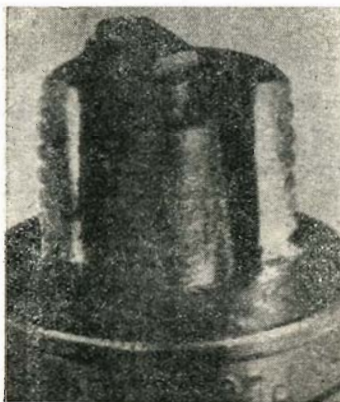
Fig. 7 - Se isolante ed elettrodi risultano ricoperti da deposito untuoso, la candela sarà « fredda », oppure — nell'eventualità che il motore abbia marciato per oltre 60.000 chilometri — la causa potrà essere imputata ai cilindri consumati e conseguenzialmente bisognosi di rettifica.
