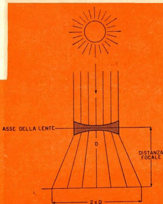
Fig. 3 - Metodo di rintraccio distanza focale per lenti negative.
