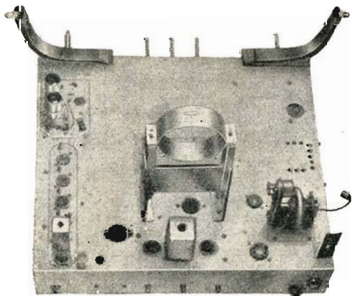
Fig. 20 - Come si presenta superiormente il telaio a montaggio meccanico ultimato
