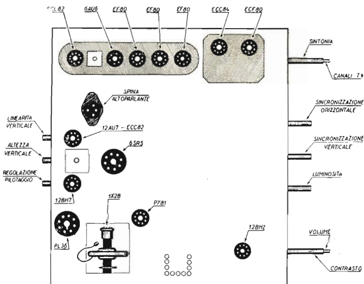
Fig. 19 - Disposizione zoccoli valvole e comandi potenziometri
