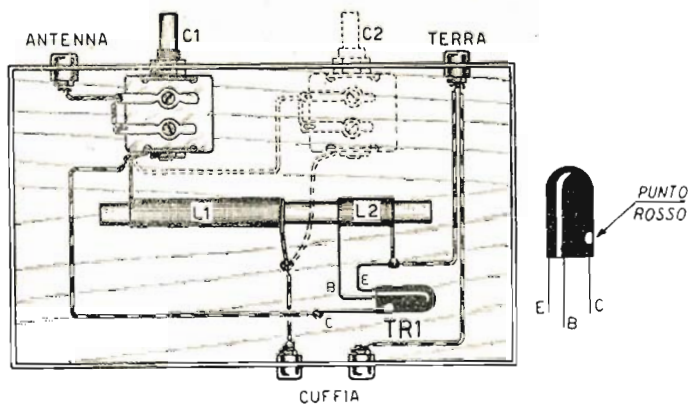
Fig. 2 - Schema pratico.
